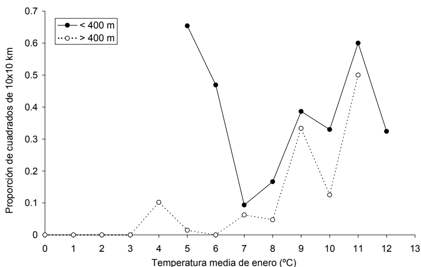
Figura 24.2. Variación de la proporción de cuadros de 10 \times 10 km donde está presente Atriplex halimus en función de la temperatura media de enero y de su altitud media.
